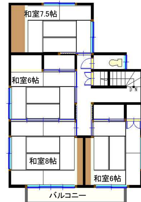
2階間取り
