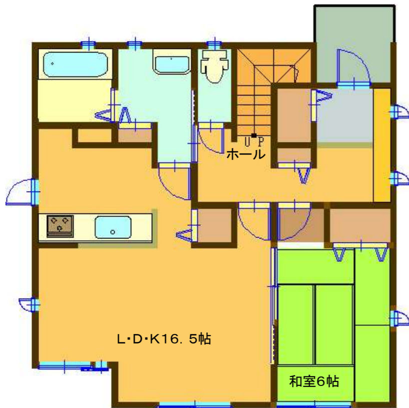
1階間取り
