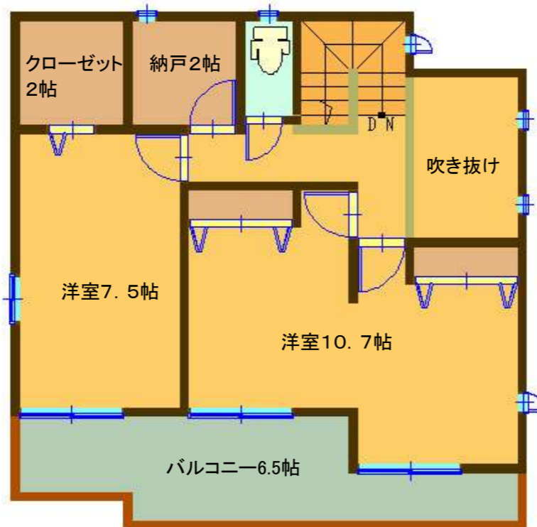
2階間取り
